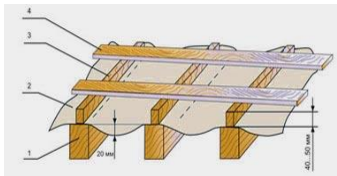
Рис.3. Укладка гидроизоляционной плёнки и обрешётки: 1 — стропильная нога; 2 — гидроизоляция; 3 — стропильная планка (брус контробрешетки); 4 — обрешётка.
