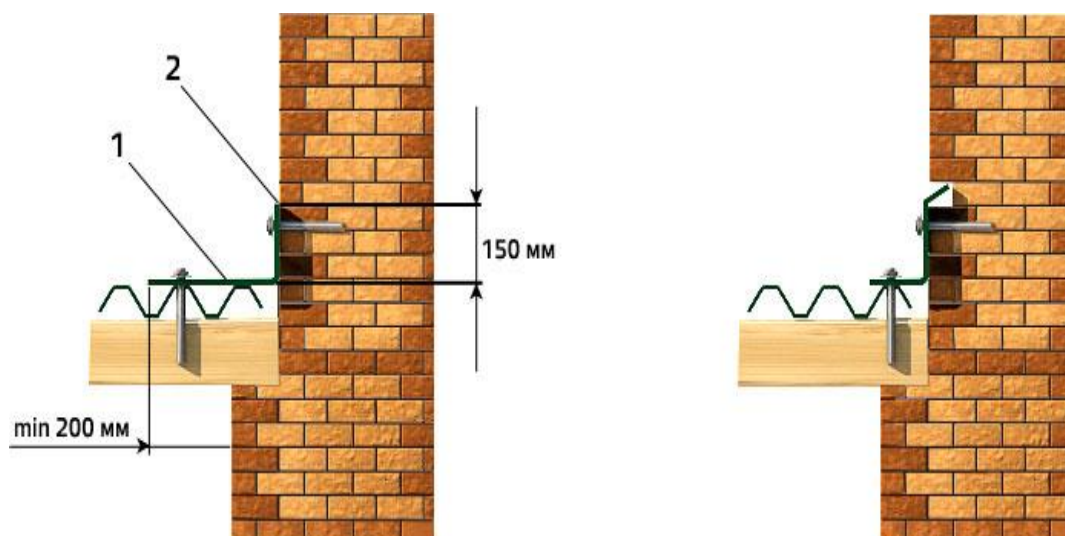
Рис.8. Поперечное примыкание ската к стене. Угловая планка при поперечном примыкании к стене крепится с шагом 200 — 300 мм и с нахлестом между планками 150 мм
