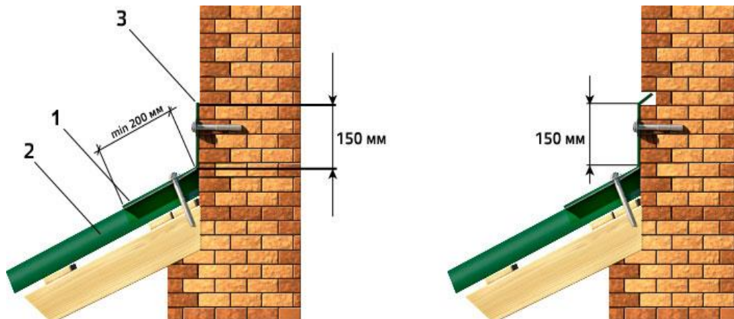
Рис.7. Продольное примыкание ската к стене. Угловая планка крепится с шагом 200 — 300 мм и с нахлестом между планками 100 — 150 мм
