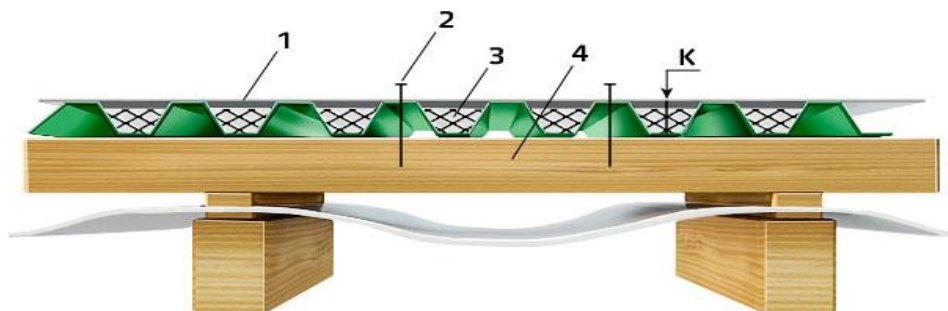
Рис.9. Крепление конька: 1 — конёк; 2 — саморез; 3 — уплотнитель коньковый; 4 — обрешётка; К — вентиляционный зазор
