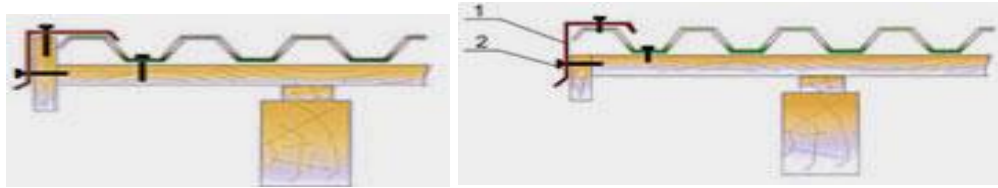
Рис.6. Крепление ветровой планки: 1 — «ветровая» планка; 2 — саморез
