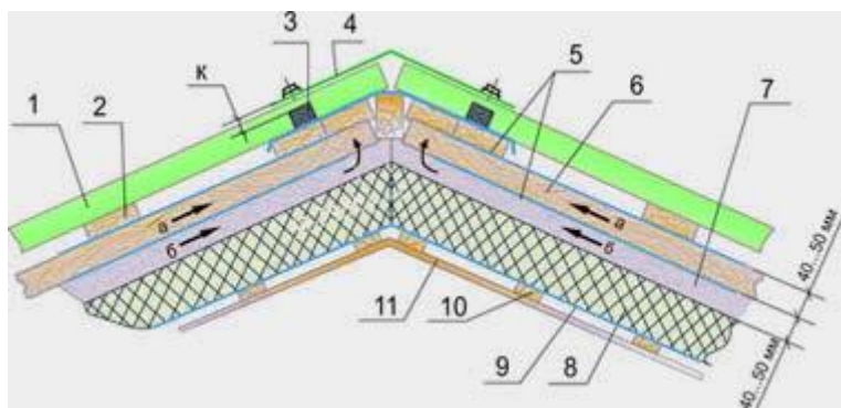
Рис.4. Утепленная кровля: 1 — профнастил (металлочерепица); 2 — обрешётка; 3 — уплотнитель коньковый; 4 — конёк; 5 — гидроизоляционная паропроницающая пленка; 6 — стропильная планка (брус контробрешетки); 7 — стропильная нога; 8 — утеплитель; 9 — паронепроницающая плёнка; 10 — потолочная рейка; 11 — гипсокартон, вагонка; а — продкровельная вентиляция; б — вентиляция между утеплителем и гидроизоляционной пленкой
