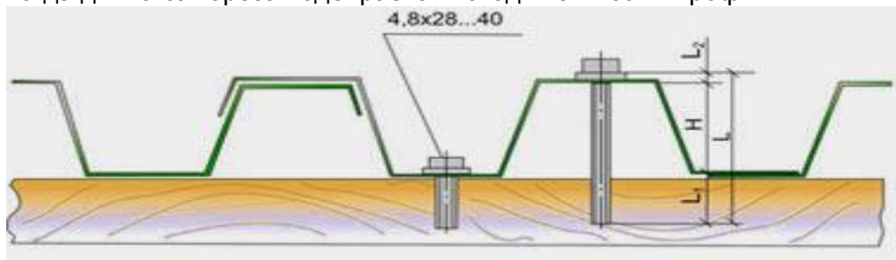
Рис.1. Крепление кровли из профнастила: L=H+L1+L2 , (мм) Где H — высота профиля профнастила, мм L1 = 25...30 мм — длина резьбовой части, которая входит в деревянную обрешетку L2 = 4 мм — толщина уплотнительной прокладки и шайбы
